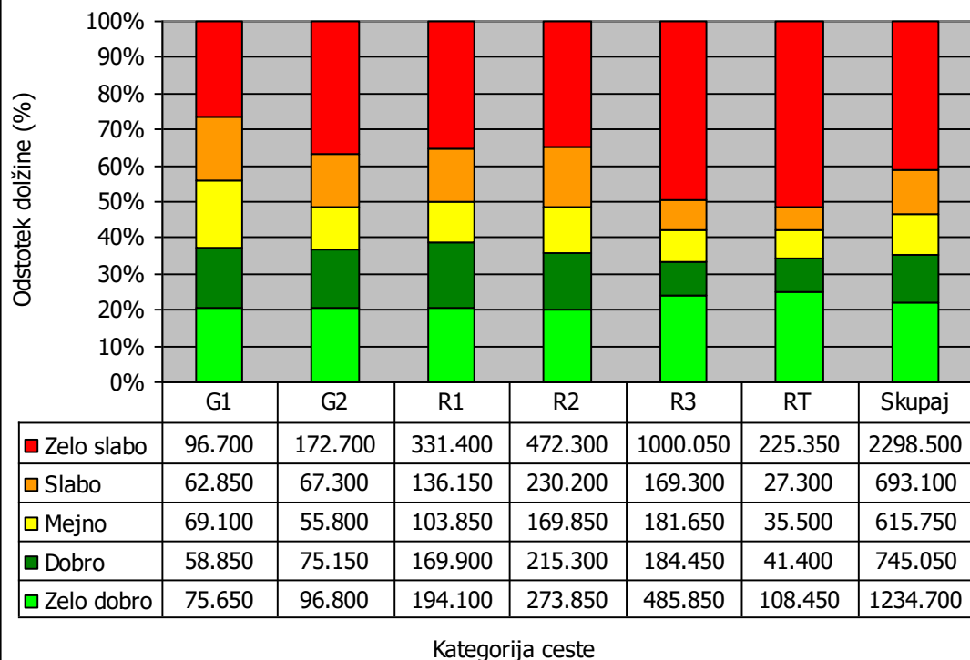
Stanje vozišč v upravljanju DRSC po vizualnem ocenjevanju v letih 2010 in 2011
